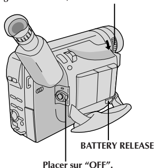
Bague d'ouverture/fermeture LENS COVER
